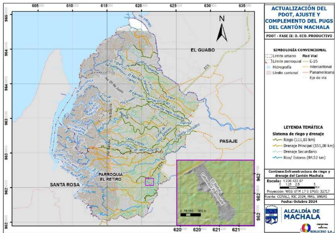
MAPA 1.62 INFRAESTRUCTURA DE RIEGO Y DRENAJE DEL CATÓN MACHALA
